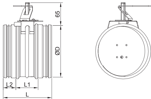
Platine de moteur, pos. haute (MH)
