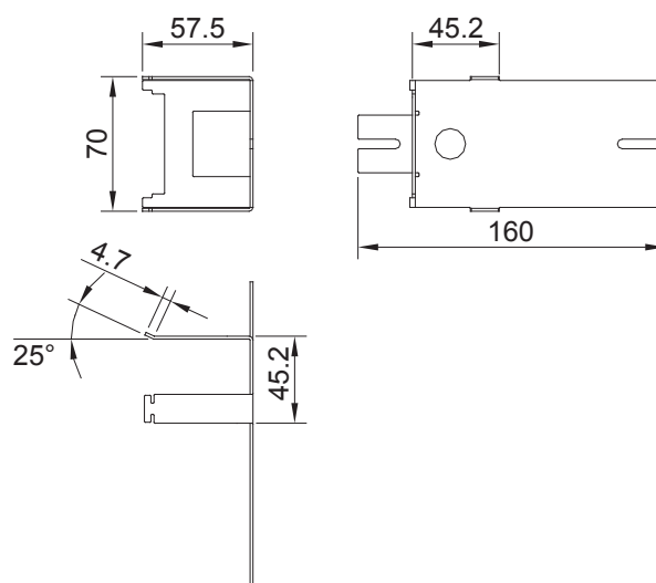
Platine de moteur, pos. haute (MH)
