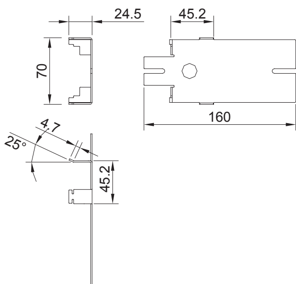
Platine de moteur, pos. basse (ML)
